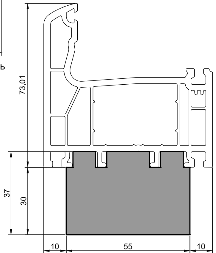
FP55-12.04 Тёплый подставочный профиль BLAUGELB 30/37X55X1200MM (Plafen S-line)
