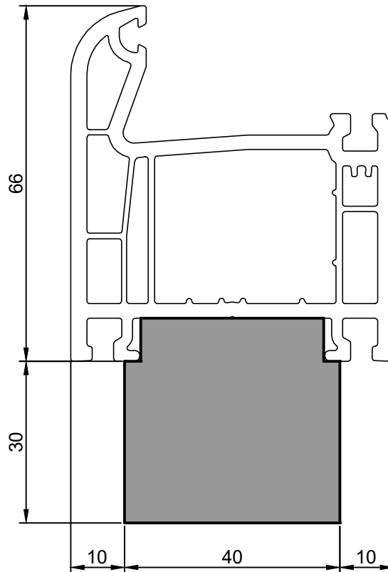
FP40-12.02 Тёплый подставочный профиль BLAUGELB 30/38X40X1200MM (Plafen E-line, L-line)
