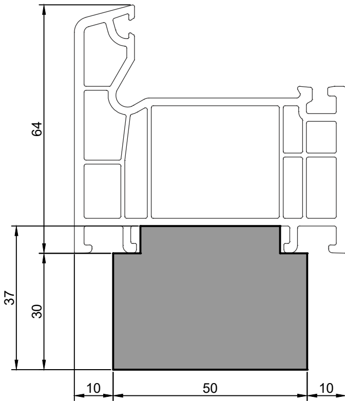
FP50-12.03 Тёплый подставочный профиль BLAUGELB 30/37X50X1200MM (Plafen T-line)
