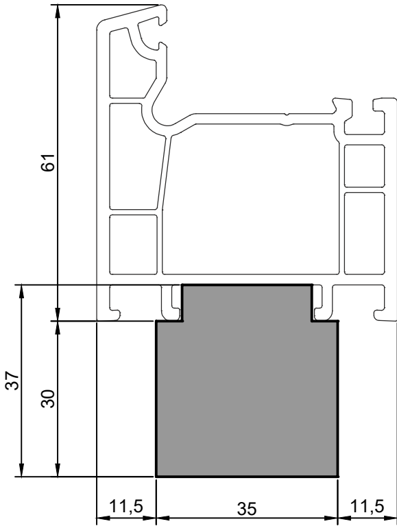
FP35-12.01 Тёплый подставочный профиль BLAUGELB 30/37X35X1200MM (Plafen C-line)
