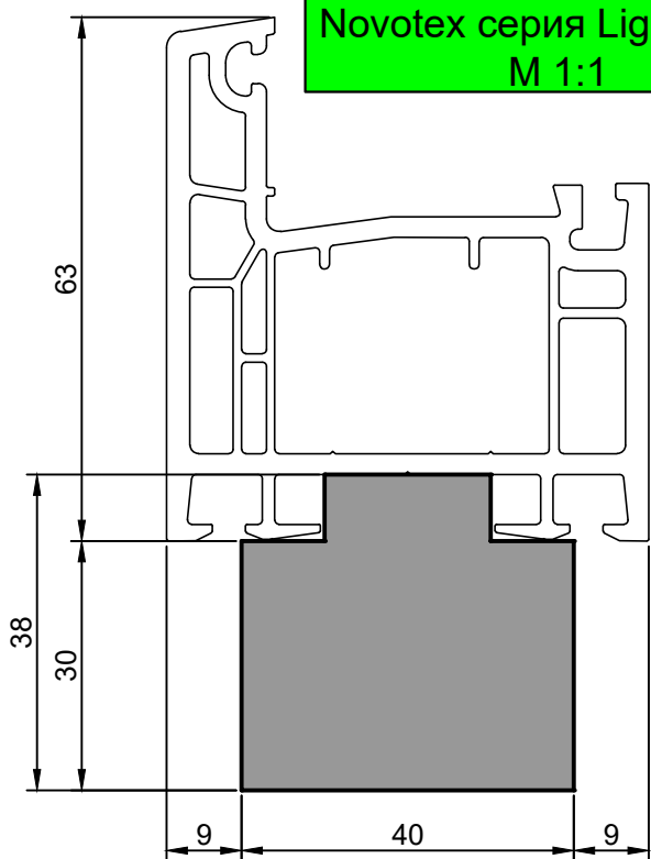
FP40-15.01 Тёплый подставочный профиль BLAUGELB 30/38X40X1200MM (Novotex Light/Classic)
