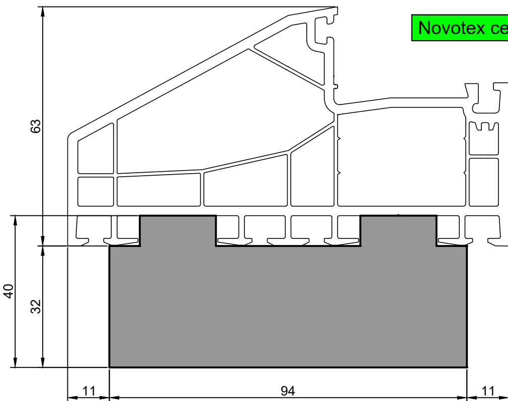
FP40-15.01 Тёплый подставочный профиль BLAUGELB 30/38X40X1200MM (Novotex Light/Classic)
