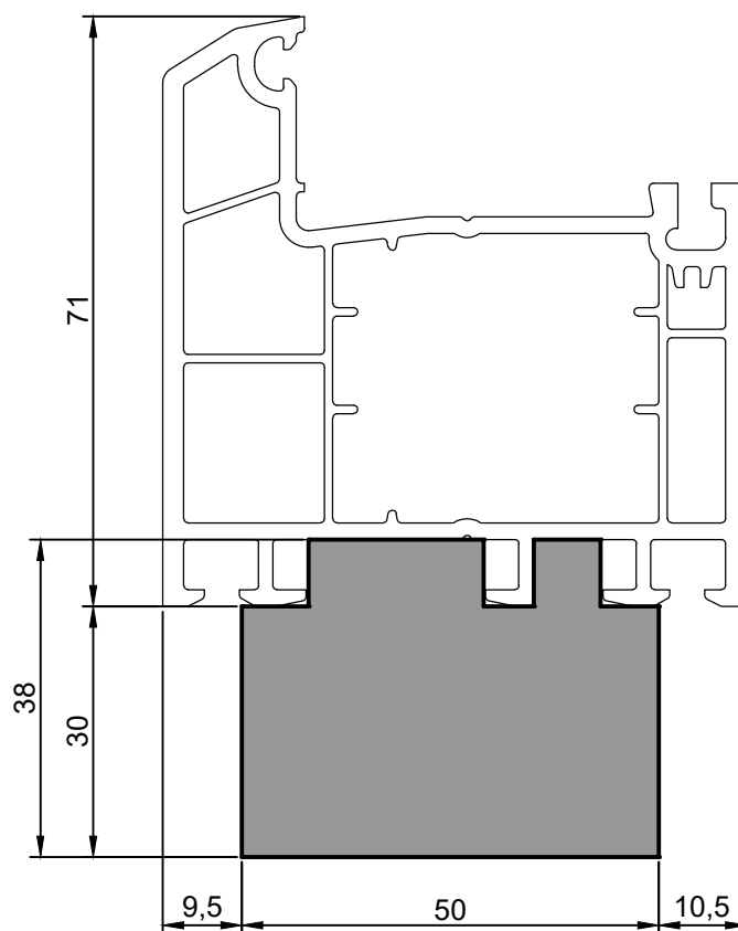
FP50-13.02 Тёплый подставочный профиль BLAUGELB 30/38X50X1200MM (Krauss 7300,7500)
