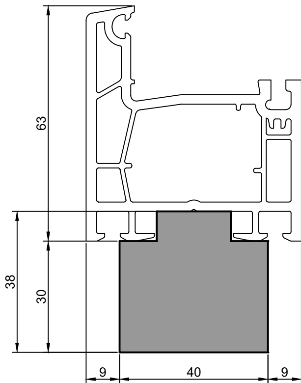
FP40-13.01 Тёплый подставочный профиль BLAUGELB 30/38X40X1200MM (Krauss 5800)
