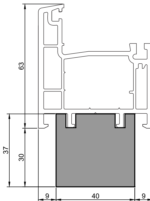
FP40-10.02 Тёплый подставочный профиль BLAUGELB 30/37X40X1200MM (PROPLEX OPTIMA, BASIS)
