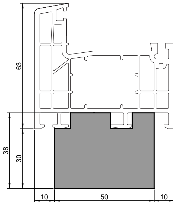
FP50-10.04 Тёплый подставочный профиль BLAUGELB 30/38X50X1200MM (PROPLEX PREMIUM, HIT)
