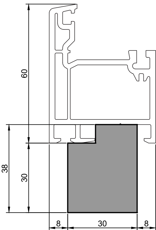
FP30-10.01 Тёплый подставочный профиль BLAUGELB 30/38X30X1200MM (PROPLEX OUT-LINE)
