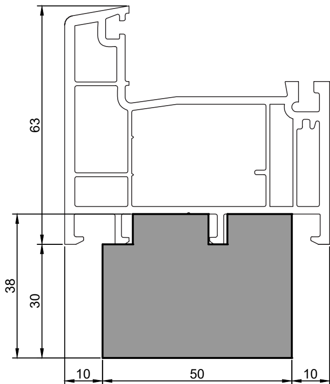
FP50-10.03 Тёплый подставочный профиль BLAUGELB 30/38X50X1200MM (PROPLEX COMFORT)
