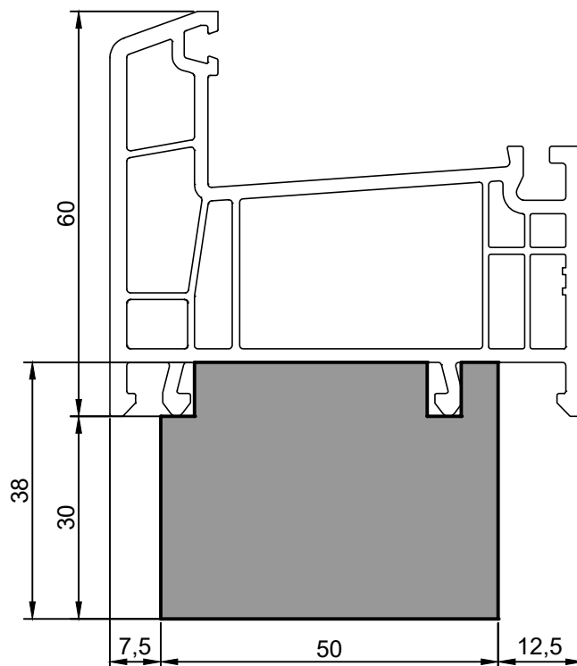
FP50-5.02 Тёплый подставочный профиль BLAUGELB 30/38X50X1200MM (Brusbox SUPER AERO)
