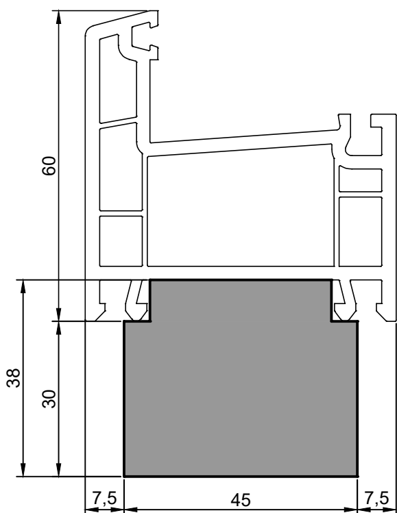
FP45-5.01 Тёплый подставочный профиль BLAUGELB 30/38X45X1200MM (Brusbox AERO / 60-3 / 60-4)
